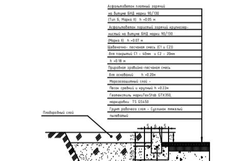
КОНСТРУКЦИЯ АСФАЛЬТОБЕТОННОГО ПРОЕЗДА
