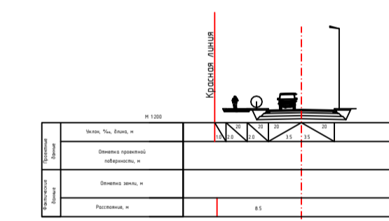
КОНСТРУКЦИЯ АСФАЛЬТОБЕТОННОГО ПРОЕЗДА
