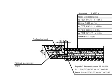
КОНСТРУКЦИЯ БРУСЧАТОГО ТРОТУАРА
