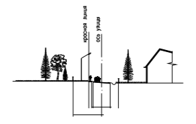
Поперечный профиль проезда на окончание улицы N 4 Разрез 15-15
