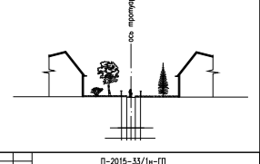
Поперечный профиль по транзитному пешеходному трамваю Разрез 8-8
