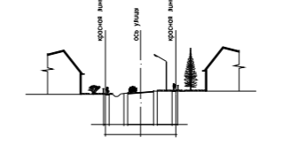
Поперечный профиль улиц NN 2, 4, 2A Разрезы 5-5, 11-11, 12-12
